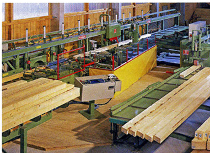
Die Abbundmaschine K1 (li. Bild), ebenso wie die P10 (re. Bild), waren Vorgängermodelle der aktuellen K2i-Anlage – beide sind heute gefragte Maschinen am Gebrauchtmarkt
